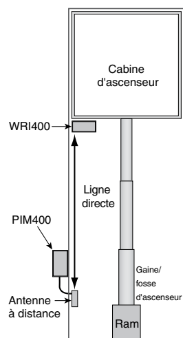
Ascenseur hydraulique
