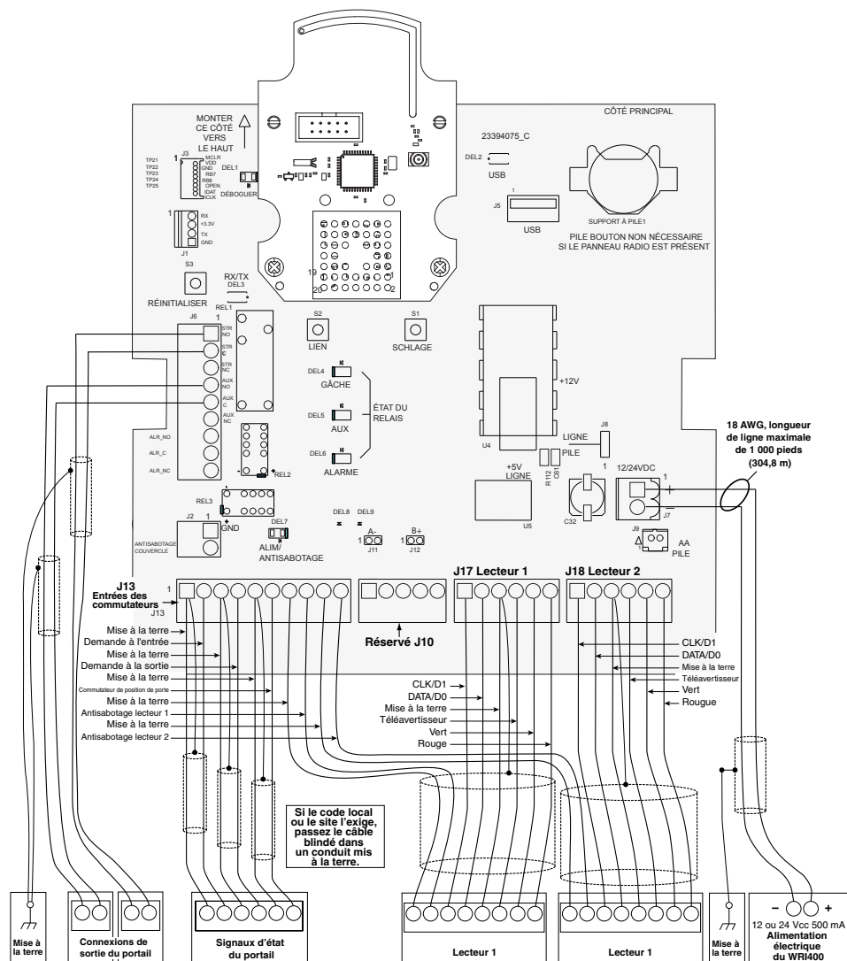
Diagramme de branchement typique du WRI400 aux lecteurs et au portail
